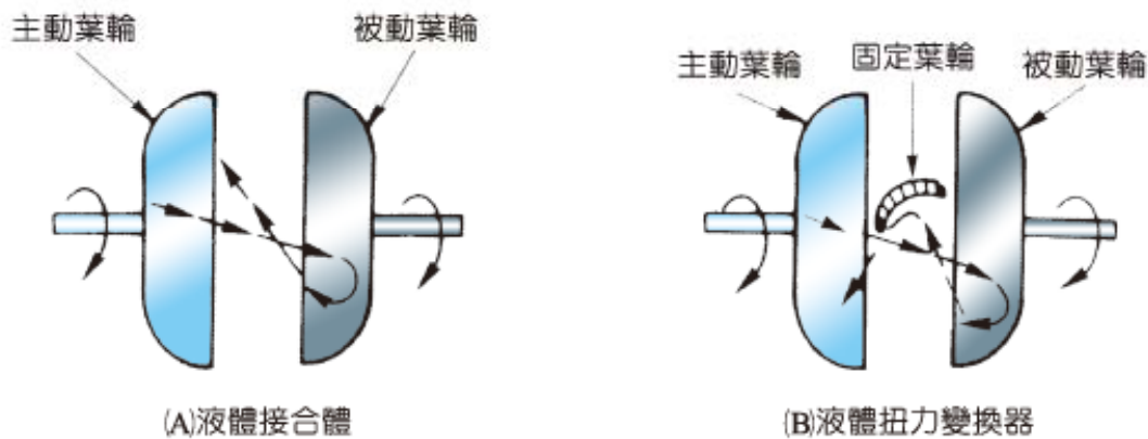
圖 2-59 在液體接合器中裝固定葉輪 (TOYOTA 修護手冊)
