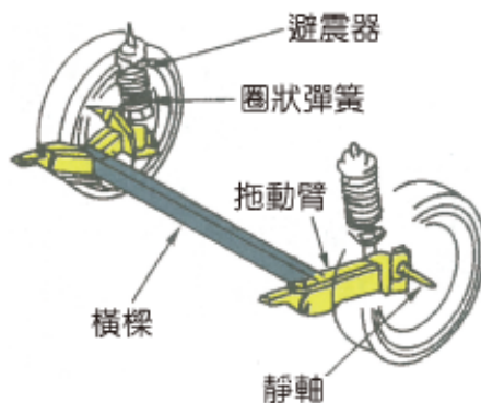
圖 2-154 前輪驅動式後軸（拖動臂式）（Automechanics fundamentals）
