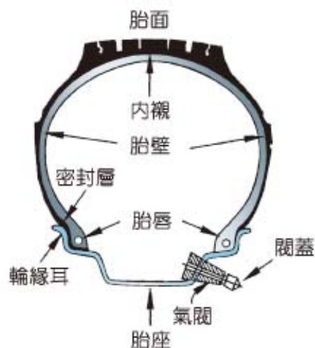
圖 5-22 無內胎輪胎 (三級自動車シャーシ)
