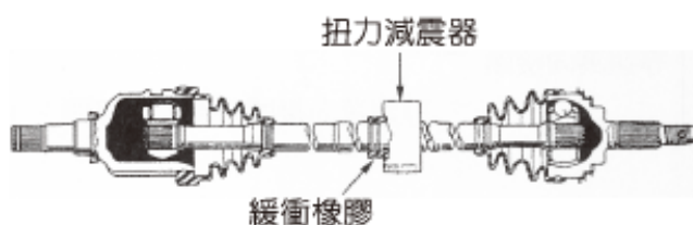
圖 2-153 扭力減震器的位置（Automechanics fundamentals）
