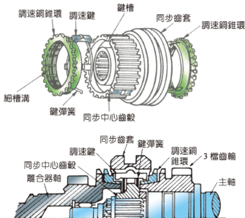
圖 2-39 鍵式同步調速裝置（四前進檔）（NISSAN 修護手冊）
