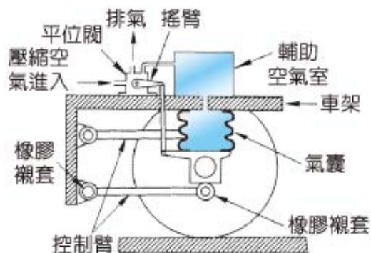
圖 3-22 空氣彈簧 (三級自動車シャーシ)
