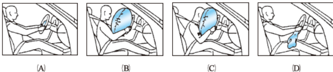
圖 7-7 SRS 之作用過程（以 50 km/h 固定壁作正面撞擊）（CIVIC 修護手冊）
