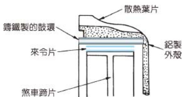
圖 6-25 鑄鐵及鋁組合式煞車鼓 (Automotive mechanics)
