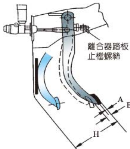
圖 2-21 離合器踏板自由行程 (NISSAN 修護手冊)
