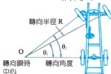
圖 4-4 轉向瞬時中心、轉向半徑及轉向角度 (自動車設計)
