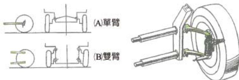
圖 3-47 拖動臂式獨立懸吊裝置 (Automechanics fundamentals)
