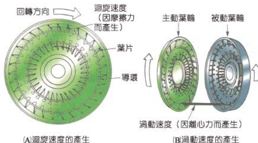
圖 2-56 液體在葉輪中之速度 (AT 車のすべて)
