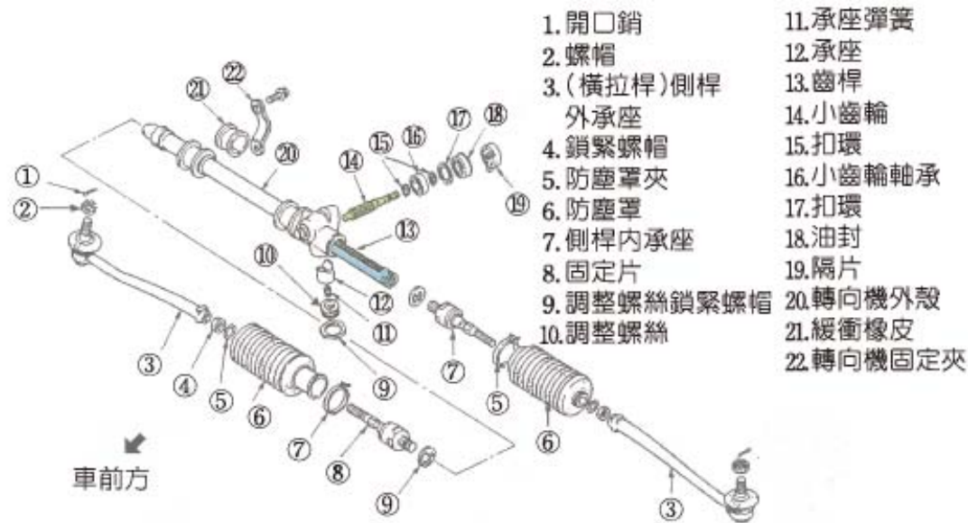
(A) RP 式轉向機分解圖
