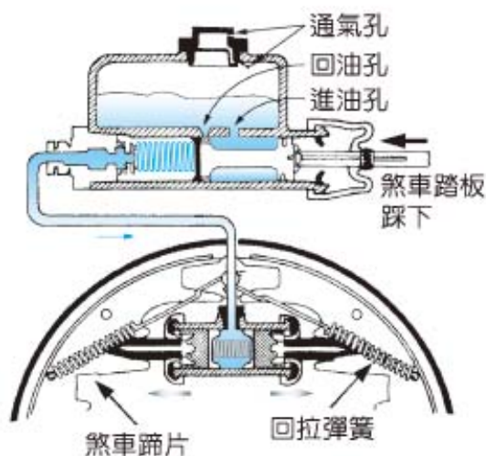
圖 6-13 煞車踏板踩下時 (Automotive handbook)
