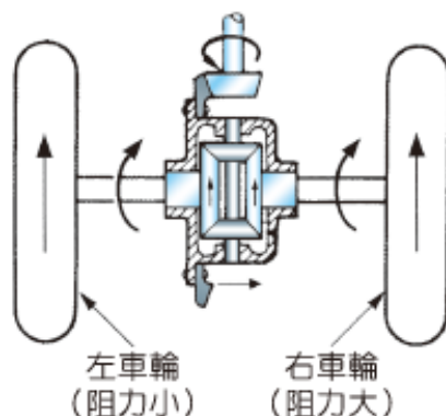
圖 2-130 車輛向右轉時差速器之作用 (自動車設計)
