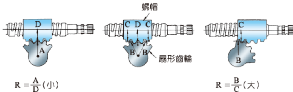
圖 4-16 RB 式轉向機之可變轉向減速比（TOYOTA 修護手冊）
