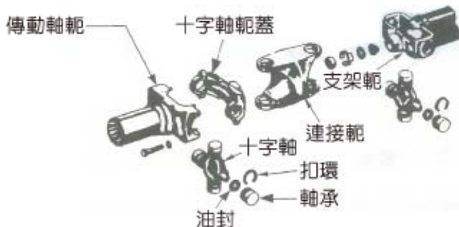
圖 2-119 雙十字軸及軛型等速萬向接頭 (現代汽車底盤)
