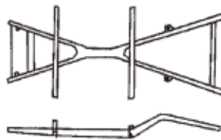
圖 3-4 X 型車架 (自動車工學)
