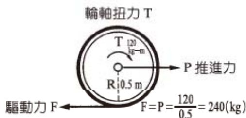
圖 2-25 扭力與驅動力的關係
