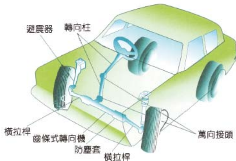
圖 1-5 轉向系統（自動車工學）
