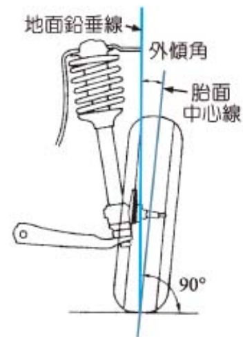
圖 4-46 外傾角 (現代汽車底盤)
