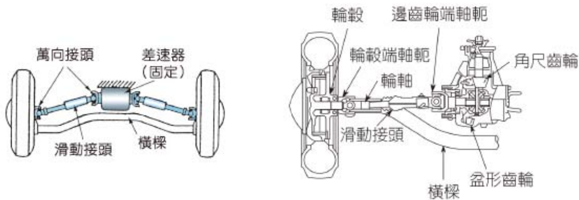
圖 2-144 擺動式後軸構造 (現代汽車底盤)
