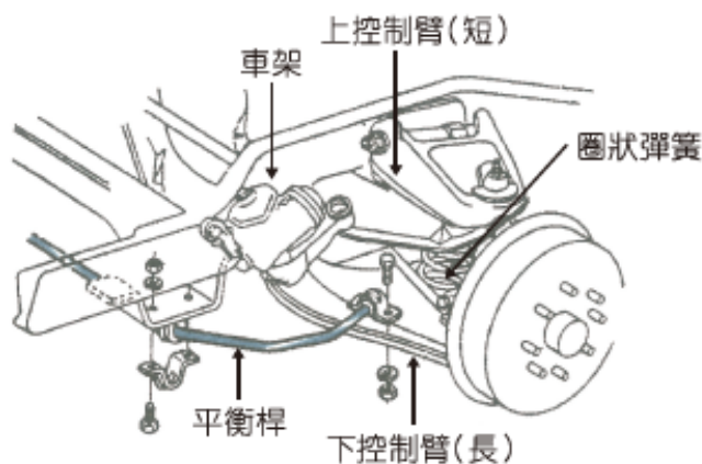
圖 3-39 平衡桿（現代汽車底盤）
