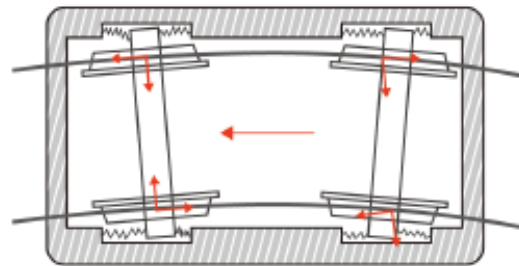
圖 8-23 徑向式轉向架（鐵道的科學）
