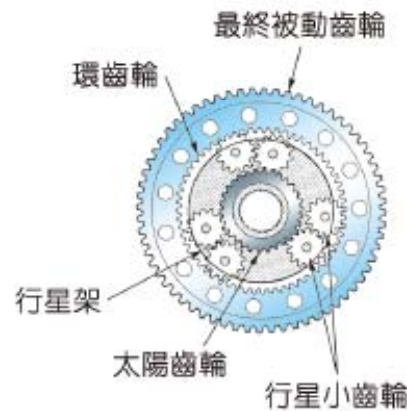
圖 2-137 ASD 之構造 (Honda) (CIVIC 修護手冊)
