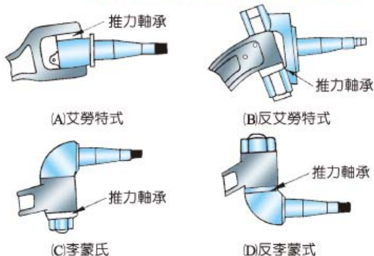
圖 3-41 整體式前軸大王銷安裝方法 (現代汽車底盤)
