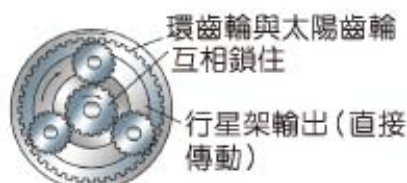
圖 2-89 “D 1 ” 檔各組件的作用 (NISSAN 修護手冊)
