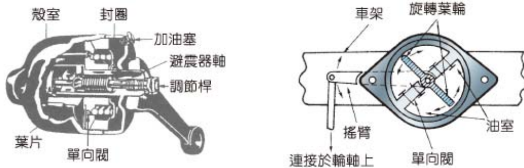
圖 3-36 轉葉型避震器（自動車工學）
