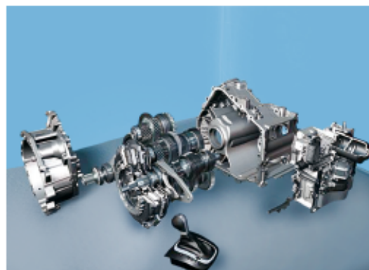
圖 2-100 AUDI DSG 6 速自、手動變速箱(U-Car)
