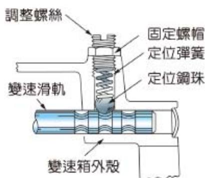
圖 2-49 定位機構 (自動車工學)
