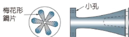
圖 6-11 煞車主缸活塞 (自動車設計)
