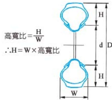
圖 5-34 輪胎直徑
