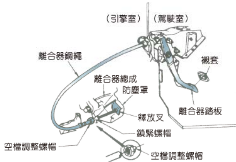
圖 2-19 鋼繩式操縱機構 (三級自動車シヤーシ)
