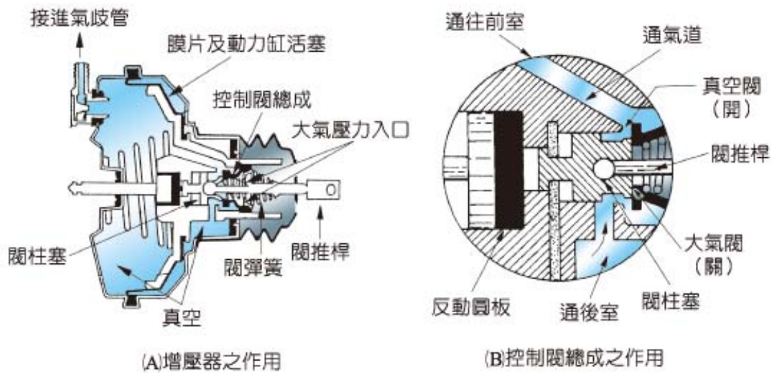
圖 6-83 引擎發動中，未踩煞車時之作用 (NISSAN 修護手冊)
