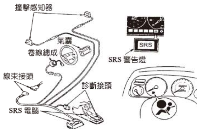
圖 7-6 SRS 組件配置圖及警告燈（CIVIC 修護手冊）
