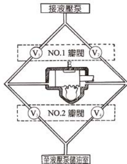
圖 4-26 閥門作動簡圖 (TOYOTA 修護手冊)
