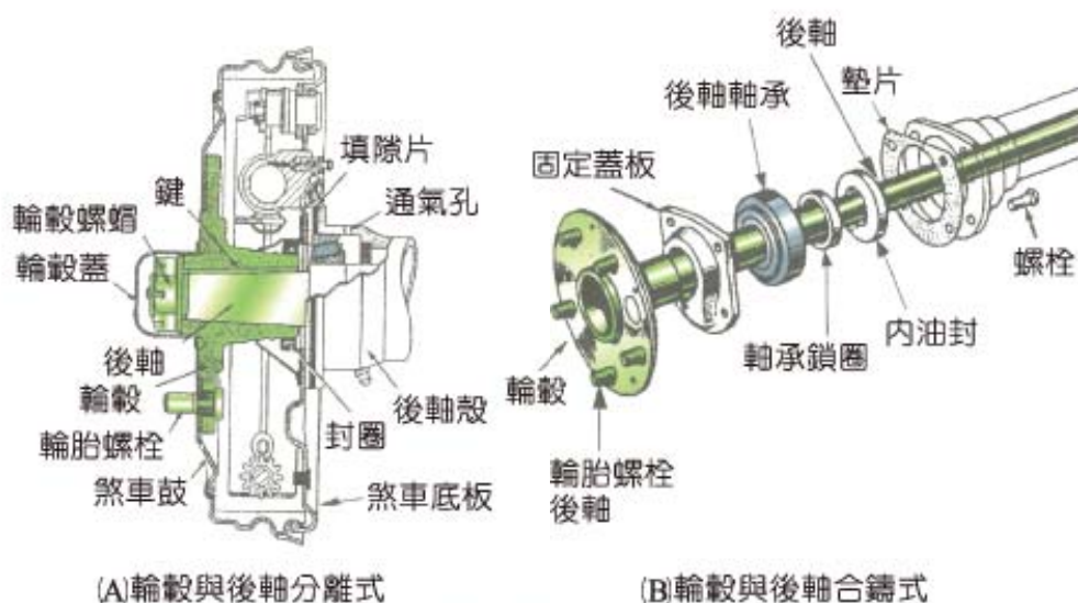
圖 5-14 半浮式後輪轂的構造 (Automotive mechanics)
