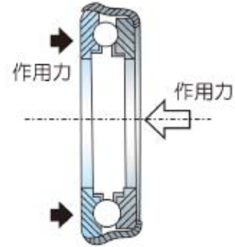
圖 2-11 釋放軸承的構造 (汽車學 2)
