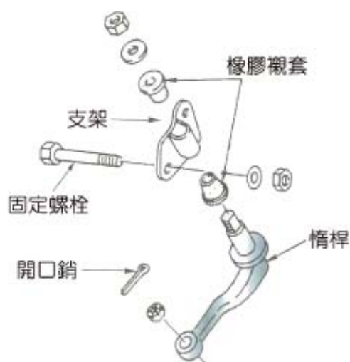
圖 4-22 惰桿總成 (NISSAN 修護手冊)
