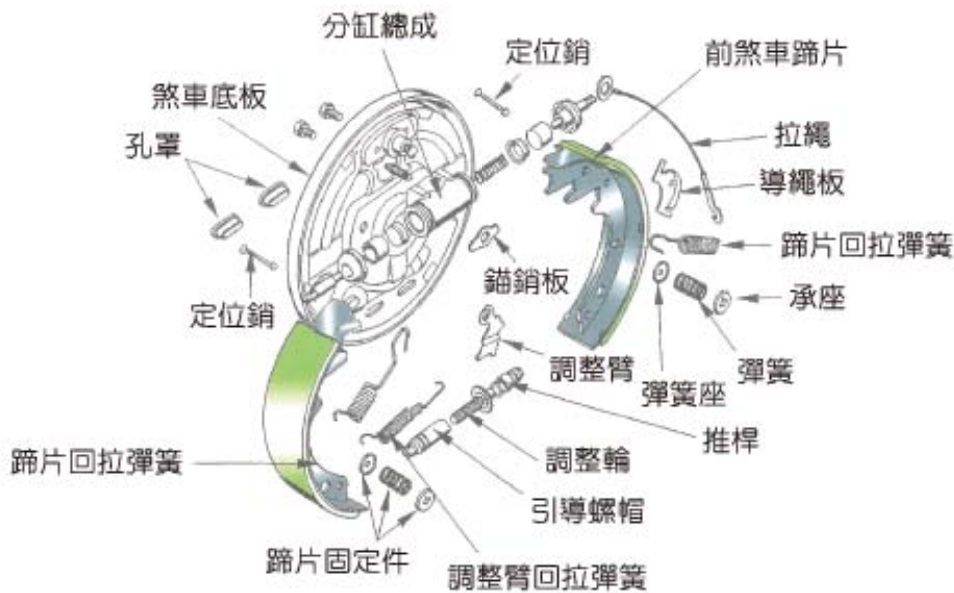
圖 6-41 本的士式腳煞車間隙自動調整分解圖 (Automotive mechanics)
