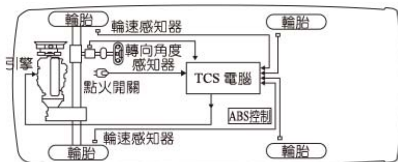
(B) TCS/ABS 配置圖
