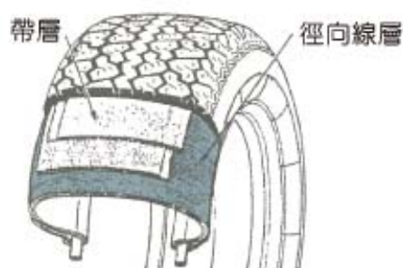
圖 5-24 徑向層輪胎 (Automechanics fundamentals)
