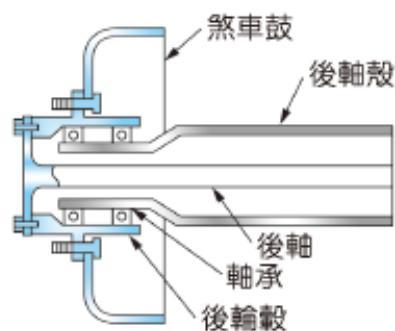
圖 2-143 全浮式後軸 (現代汽車底盤)
