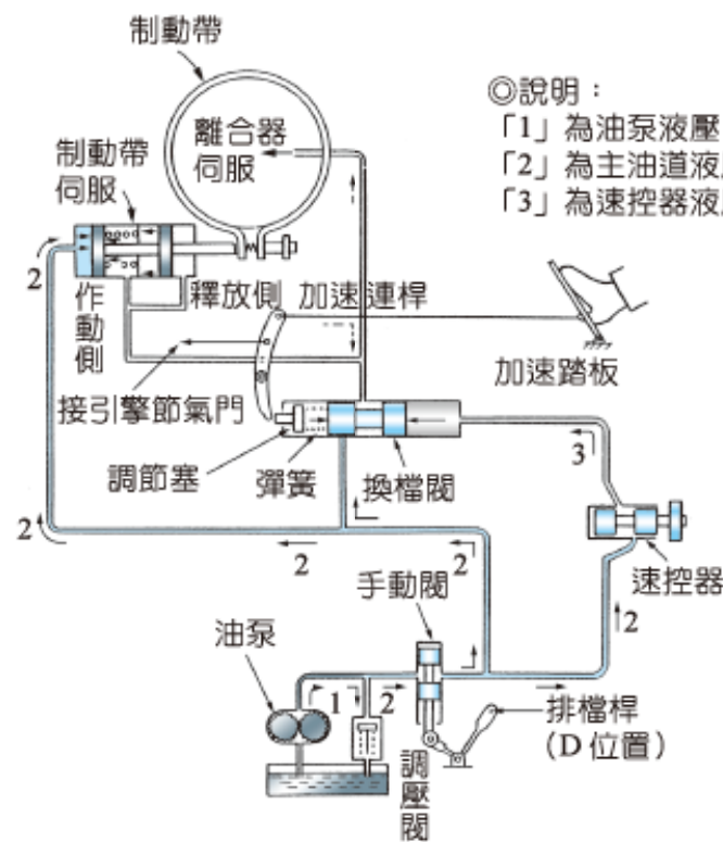
圖 2-80 自動換檔作用整體配置圖(改良)(AT車のすべて)
