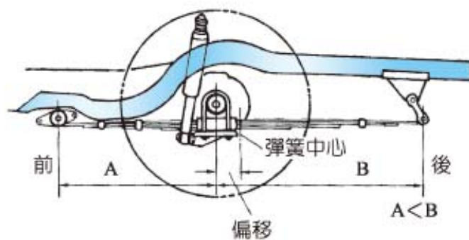
圖 3-15 非對稱型片狀彈簧 (汽車之整修與故障排除)
