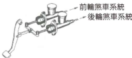
圖 6-55 並列式煞車主缸（現代汽車底盤）
