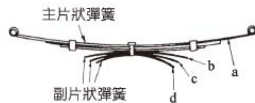
圖 3-13 多段式片狀彈簧 (自動車設計)
