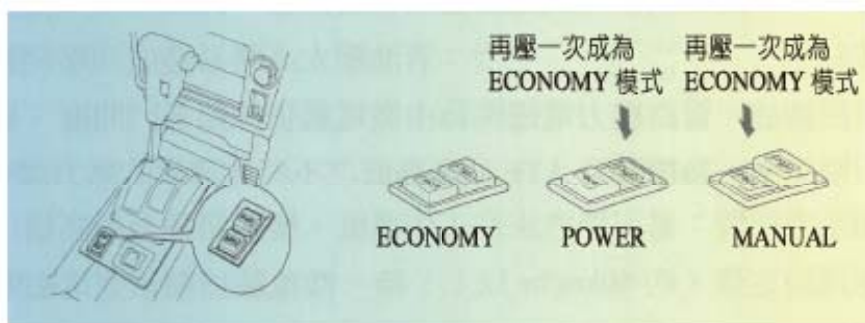
圖 2-95 模式選擇開關的位置 (AT 車的變速箱) (Automechanics fundamentals)
