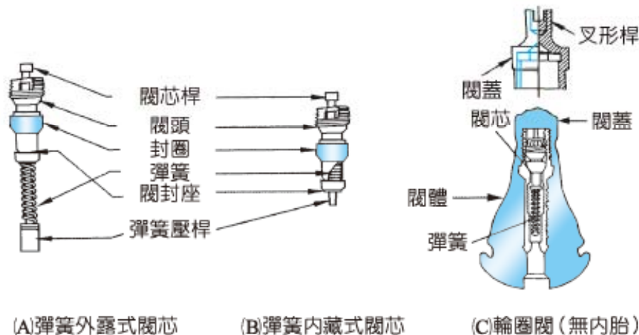
圖 5-20 氣閥與閥蓋之構造 (三級自動車シャーシ)
