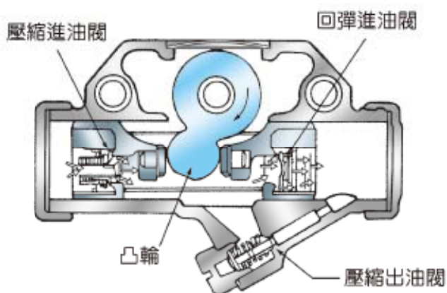
圖 3-34 搖臂活塞型單作用避震器 (彈簧壓縮時) (自動車設計)
