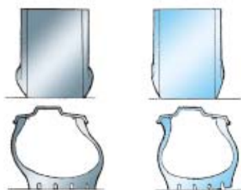
(A) 徑向層輪胎 (B) 交叉層輪胎
