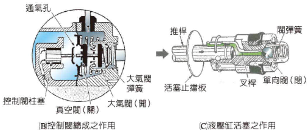
圖 6-89 煞車踏板踏下時真空增壓煞車的作用（自動車設計）
