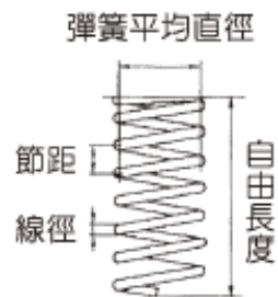
圖 3-16 圈狀彈簧 (自動車設計)
