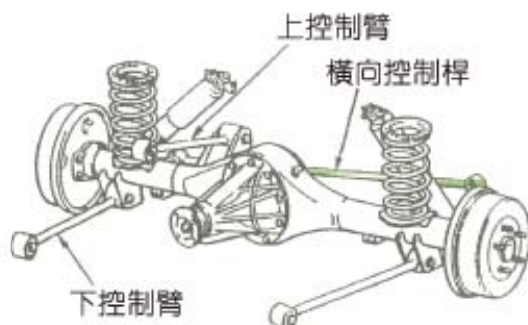
圖 3-43 橫向控制桿（偏斜桿）（現代汽車底盤）
