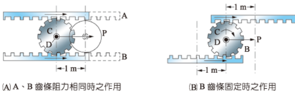
圖 2-127 差速齒輪原理（現代汽車底盤）
