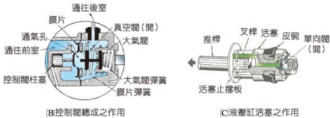
圖 6-88 煞車踏板未踩時真空液壓煞車增壓器的作用（自動車設計）
