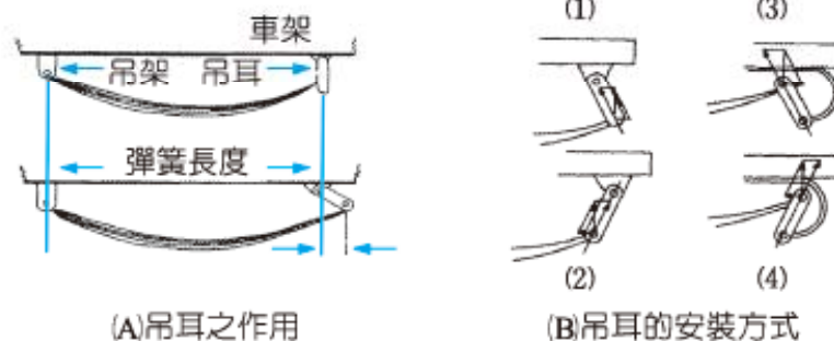
圖 3-10 片狀彈簧變形時之長度變化 (吊耳的作用) (Automotive mechanics)
