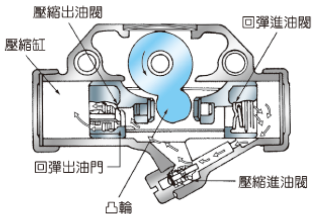
圖 3-35 搖臂活塞型單作用避震器 (彈簧反彈時) (自動車設計)
