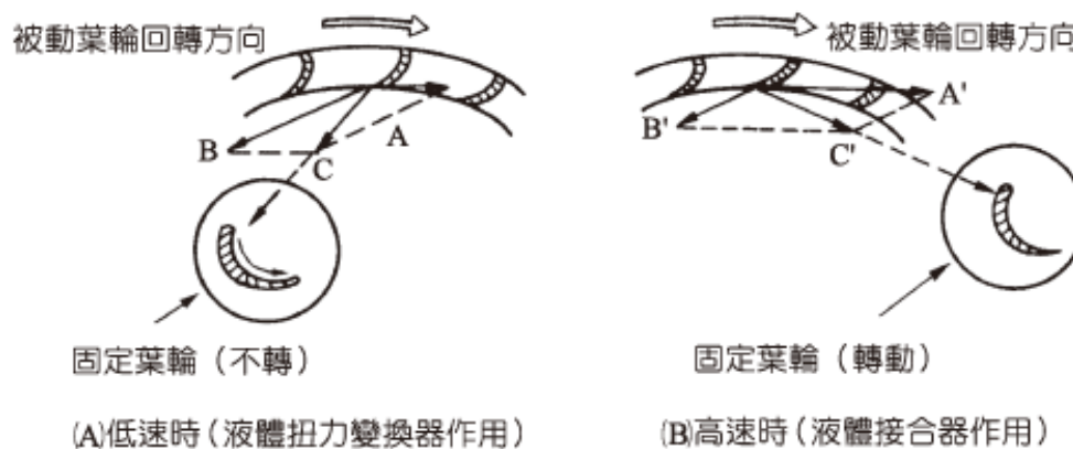
圖 2-61 液體扭力變換接合器之作用原理 (NISSAN 修護手冊)
