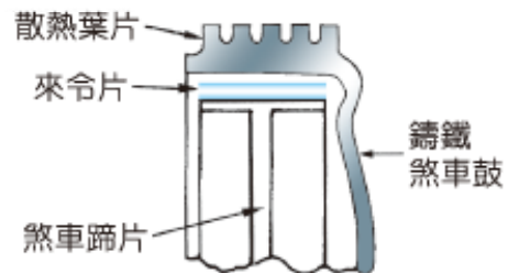
圖 6-22 鑄鐵煞車鼓 (Automotive mechanics)
