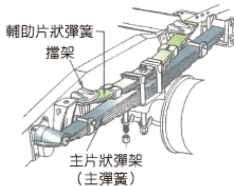
圖 3-12 兩段式片狀彈簧 (汽車學 2)
