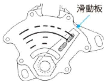
圖 2-97 空檔起動開關的構造及作用 (CIVIC 修護手冊)
