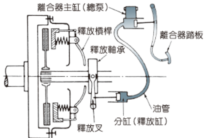
圖 2-20 液壓操縱式 (NISSAN 修護手冊)
