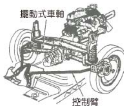
圖 3-48 擺動車軸式獨立懸吊裝置 (汽車學 2)
