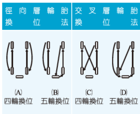
圖 5-40 輪胎換位
