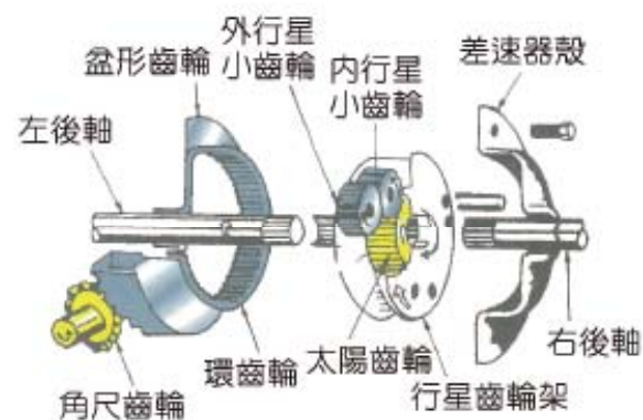
圖 2-134 行星齒輪式差速器 (三級自動車シャーシ)
