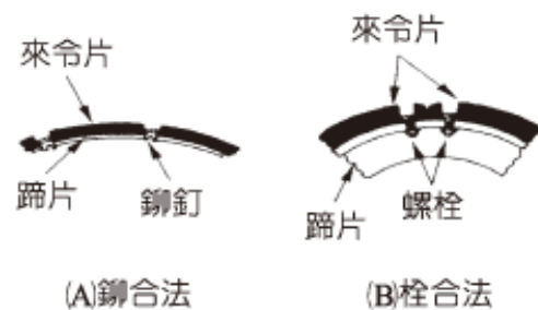
圖 6-29 鉚釘或螺栓接合之煞車來令片
