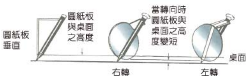
圖 4-48 內傾角自動回復的作用（汽車學 2）
