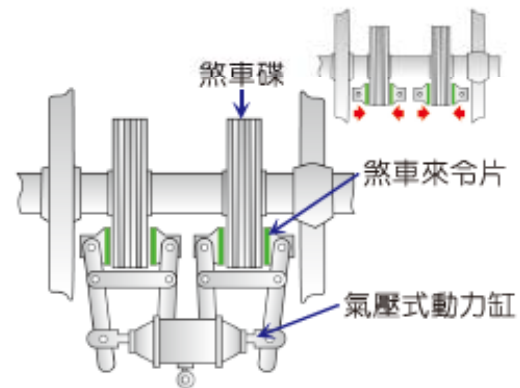
(B)構造圖
