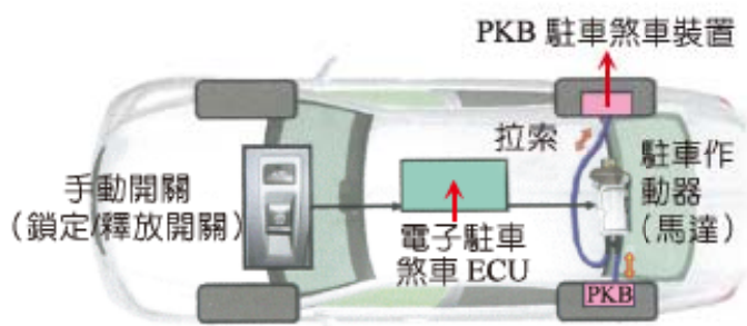
圖 6-66 鋼索牽引式 EPB 配置圖 (網路-癮科技)
