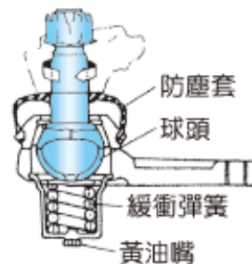
(B)球接頭的構造 (橫拉桿)
