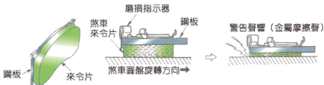
(A) 煞車來令片構造 (B) 煞車來令片新品時之作用 (C) 煞車來令片磨損時之警告作用
