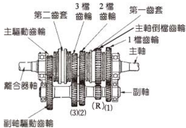
圖 2-38 鍵式同步式手動變速箱的構造 (NISSAN 修護手冊)
