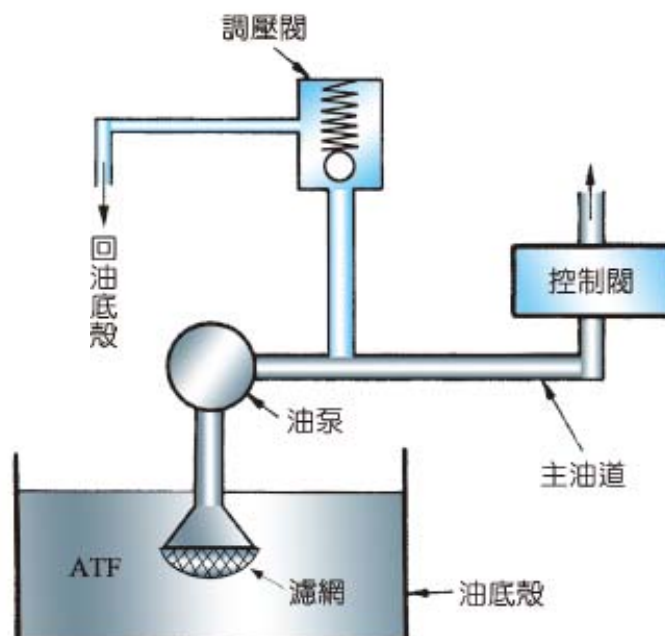
圖 2-75 調壓閥
