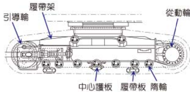
(A)履帶式挖土機
