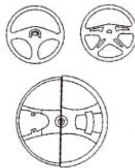
圖 4-7 方向盤內部構造（CIVIC 修護手冊）
