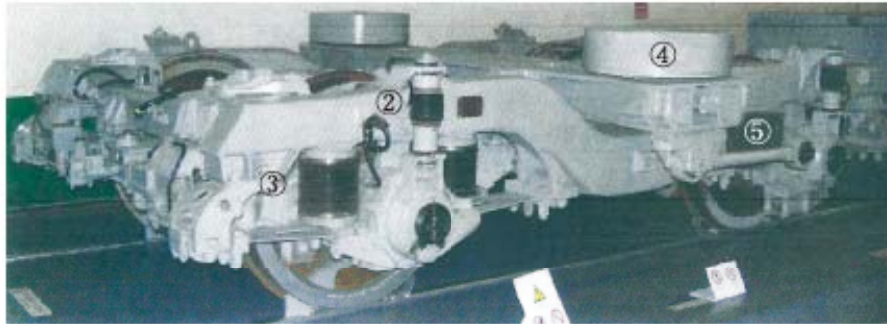
①轉向架框 ②減震器 ③初級懸掛 ④次級懸掛 ⑤扭力桿 ⑥驅動馬達 ⑦最終齒輪
