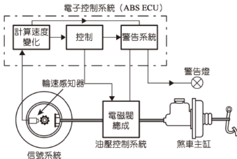
圖 6-75 NISSAN ABS 作用流程圖 (NISSAN 修護手冊)
