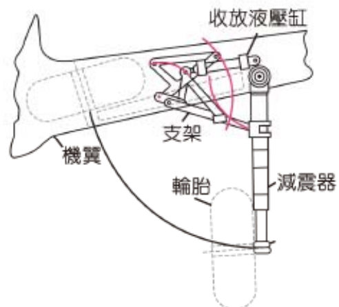
(B) 機翼輔助輪之構造
