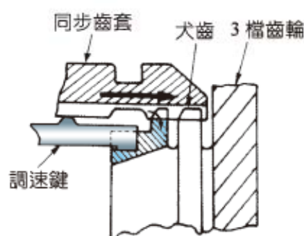
圖 2-42 調速作用 3 (NISSAN 修護手冊)
