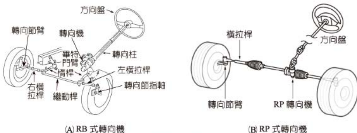
圖 4-6 獨立式前輪懸吊之轉向系統（汽車學 2）
