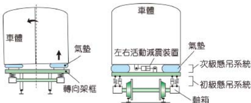
圖 8-28 氣墊式次級懸吊（鐵道的科學）
