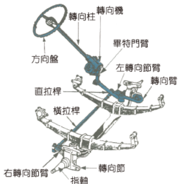
圖 4-5 整體式懸吊之轉向系統 (汽車學 2)
