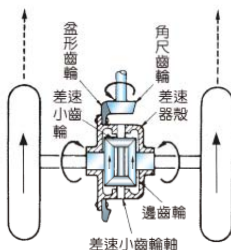
圖 2-129 直線前進時差速器之作用 (自動車設計)
