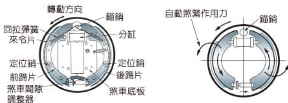
圖 6-35 雙伺服輪煞車的構造 (ブレーキ)
