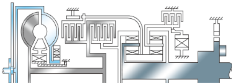
圖 2-87 “N” 檔各組件的作用 (NISSAN 修護手冊)
