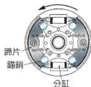
圖 6-36 複動雙引導式蹄片安裝法 (ブレーキ)
