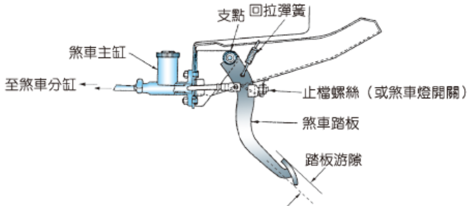
圖 6-7 掛式煞車踏板（プリーキ）
