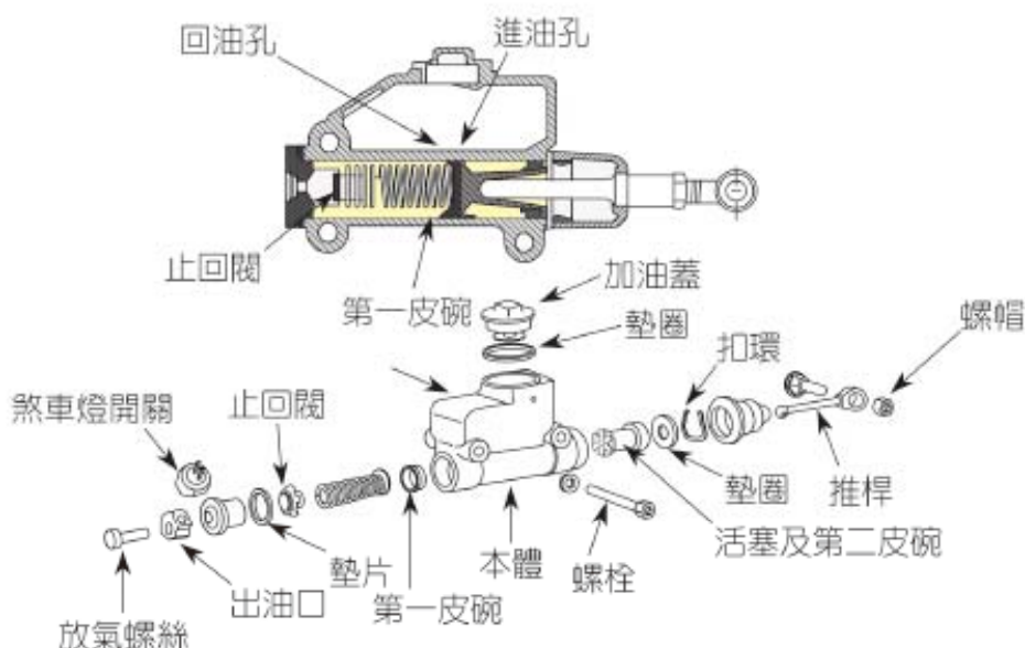
圖 6-10 煞車主缸的構造 (Automotive mechanics)
