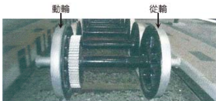
圖 8-25 車輪組（鐵道科學完全探索）
