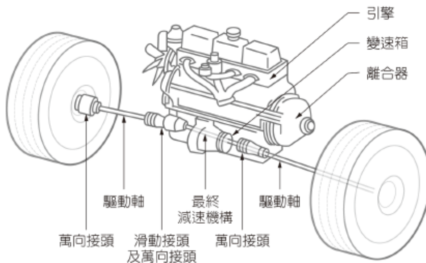
圖 2-2 前輪驅動
