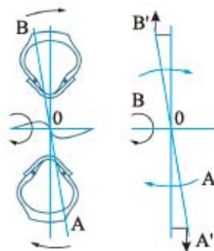
圖 5-38 動平衡不良之影響
