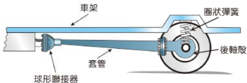
圖 2-149 套管式車輛推進 (自動車工學)
