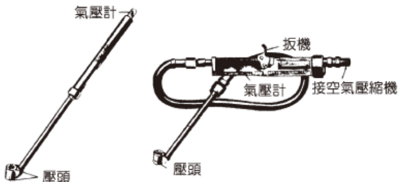
圖 5-21 輪胎氣壓計 (自動車設計)
