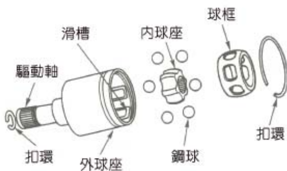
圖 2-116 雙偏位型等速萬向接頭 (三級自動車シャーシ)
