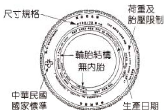
圖 5-28 輪胎側壁之各項標記（自動車工學）
