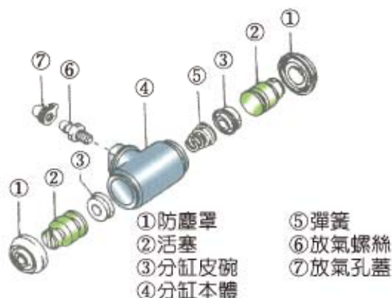
圖 6-18 煞車分缸之構造 (自動車工學)
