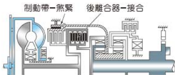
圖 2-89 “D 1 ” 檔各組件的作用 (NISSAN 修護手冊)
