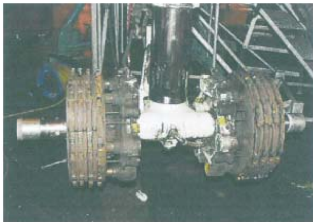
圖 8-8 多碟式煞車裝置（航空器概論）
