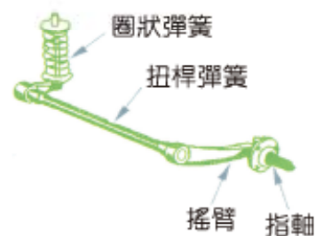
圖 3-20 扭桿與圈狀彈簧之複合彈簧 (三級自動車シャーシ)
