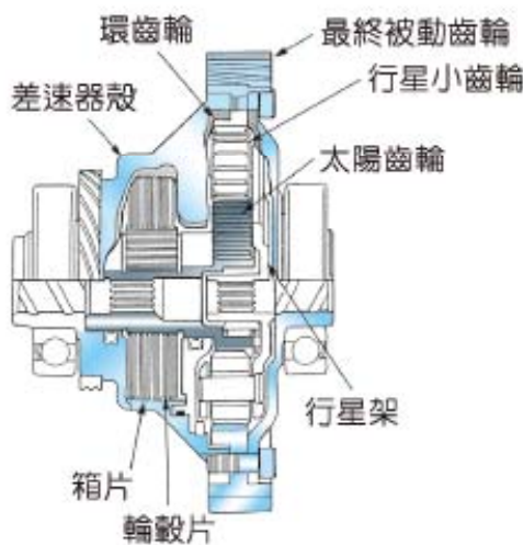
圖 2-137 ASD 之構造 (Honda) (CIVIC 修護手冊)
