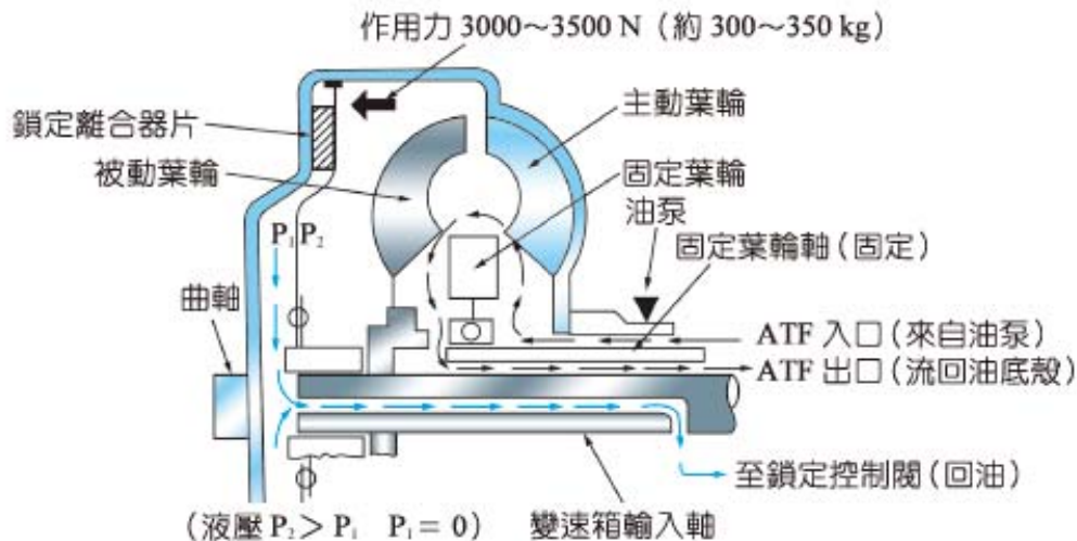
圖 2-65 鎖定制液體扭力變換接合器之作用（鎖定狀態）（三級自動車シャーシ）
