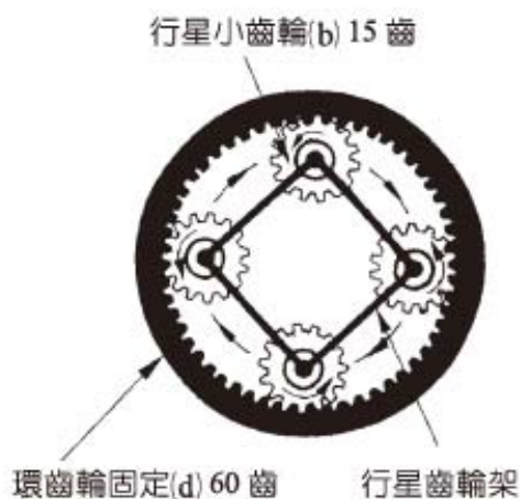
圖 2-67 行星小齒輪繞環齒輪一周
