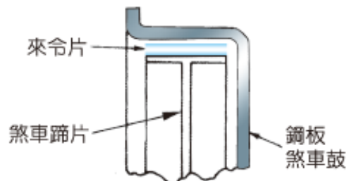
圖 6-23 鋼板煞車鼓 (Automotive mechanics)
