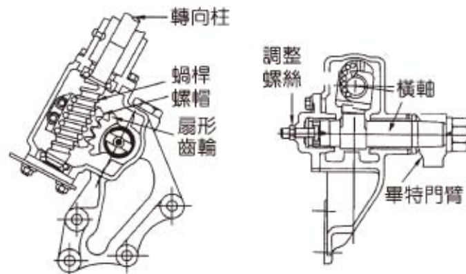
圖 4-14 (B) 循環滾珠螺帽式轉向機的剖面構造 (TOYOTA 修護手冊)
