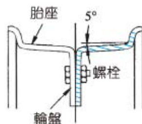
圖 5-6 分離式胎座（汽車學 2）
