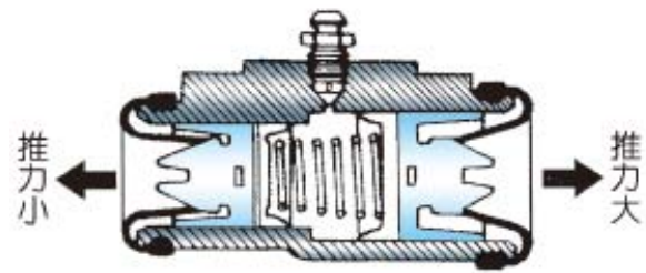
圖 6-21 級式分缸（自動車工學）
