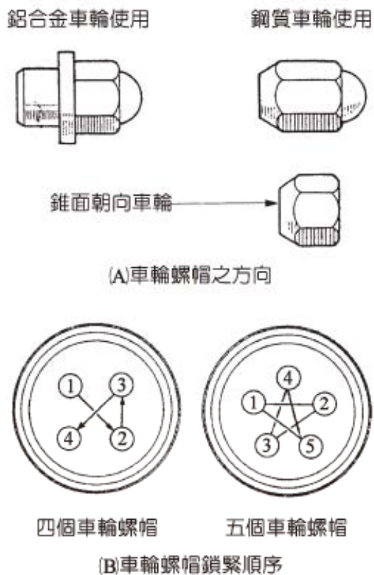
圖 5-42 車輪螺帽及鎖緊順序 (NISSAN 修護手冊)
