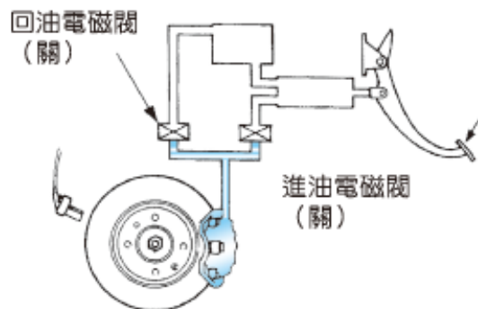
圖 6-71 ABS 之定壓控制 (ブレーキ)
