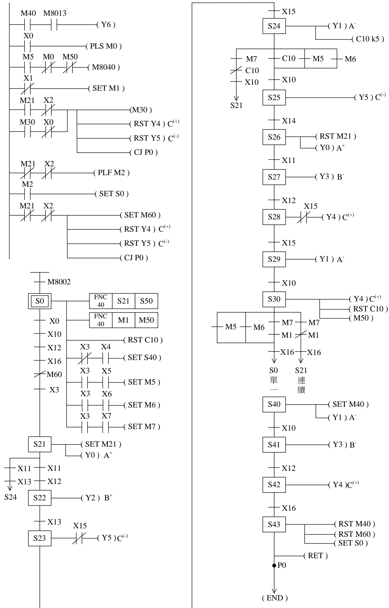
圖2-40 模式b SFC圖
