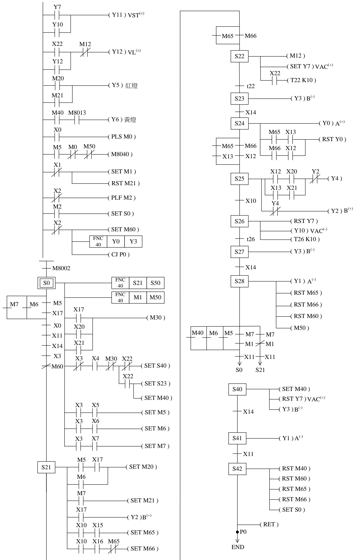
圖3-24 模式a SFC圖
