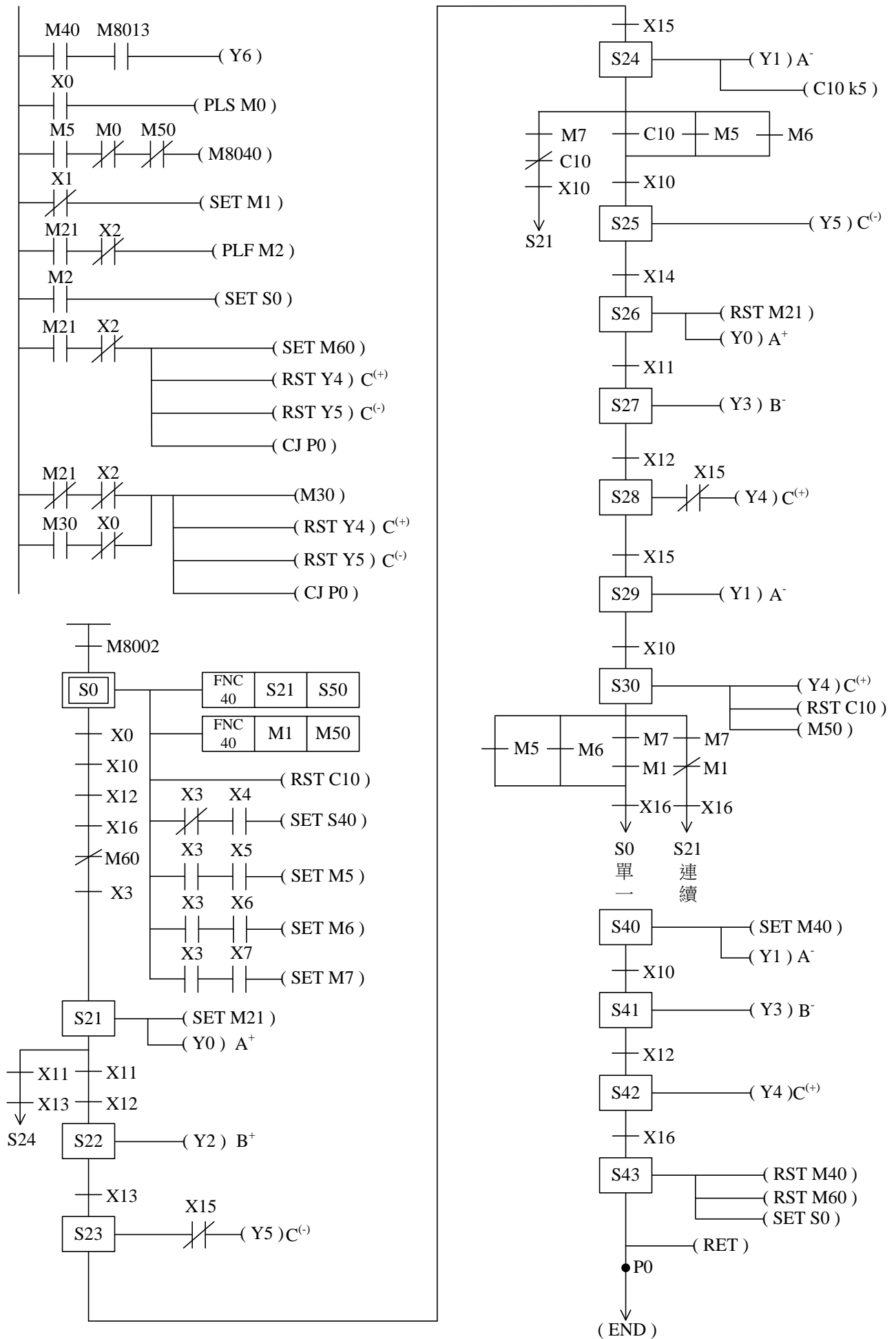
圖2-20 模式a SFC圖
