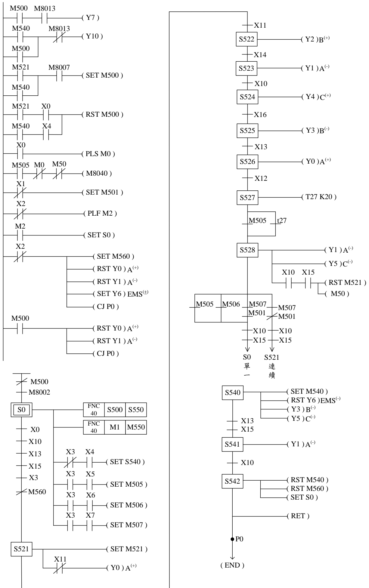
圖6-18 模式a SFC圖
