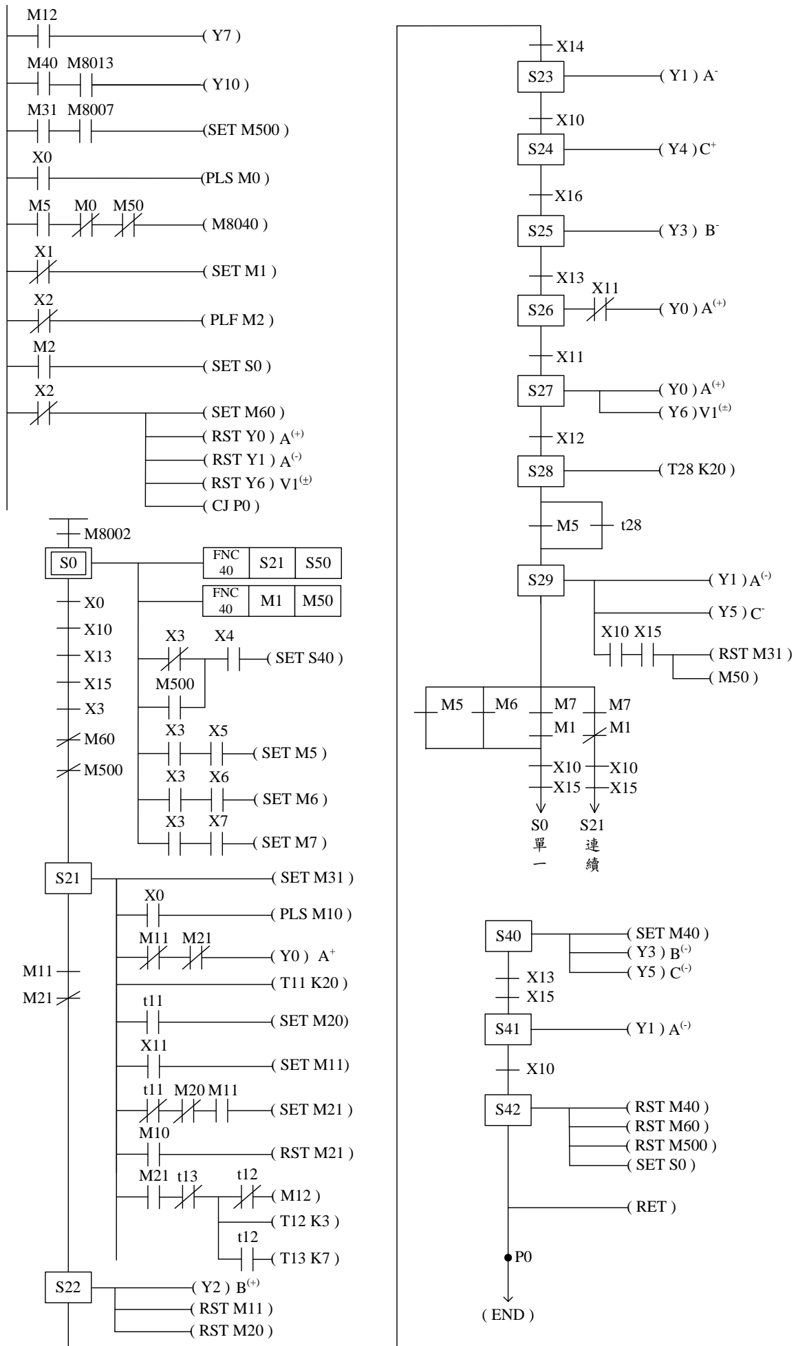
圖5-18 模式a SFC圖
