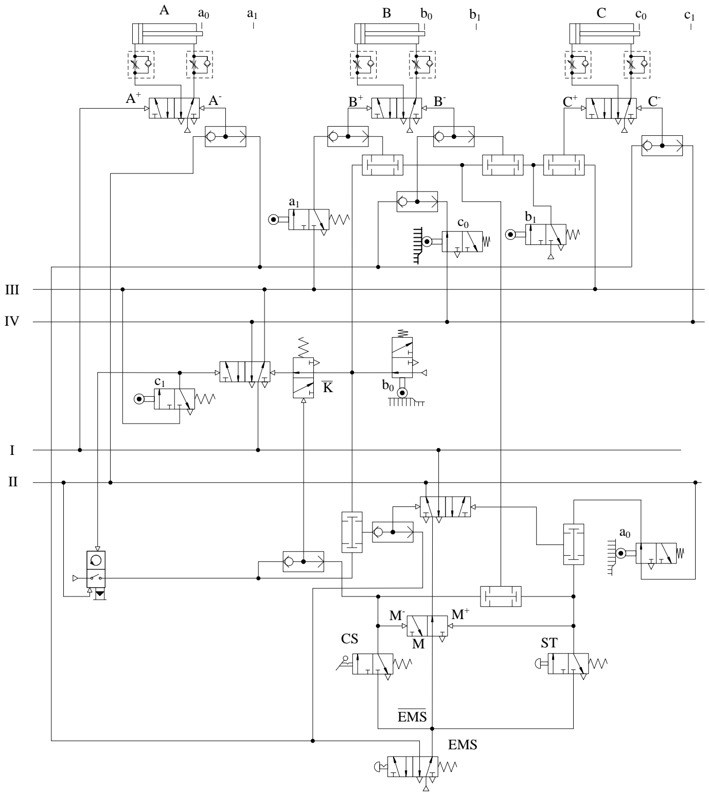
圖9-5 計數反覆動作回路
