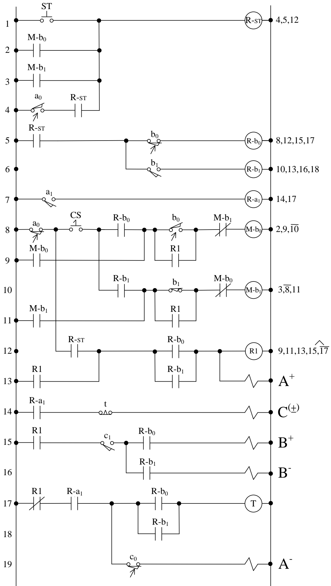
圖8-3b 電路圖(另解)
