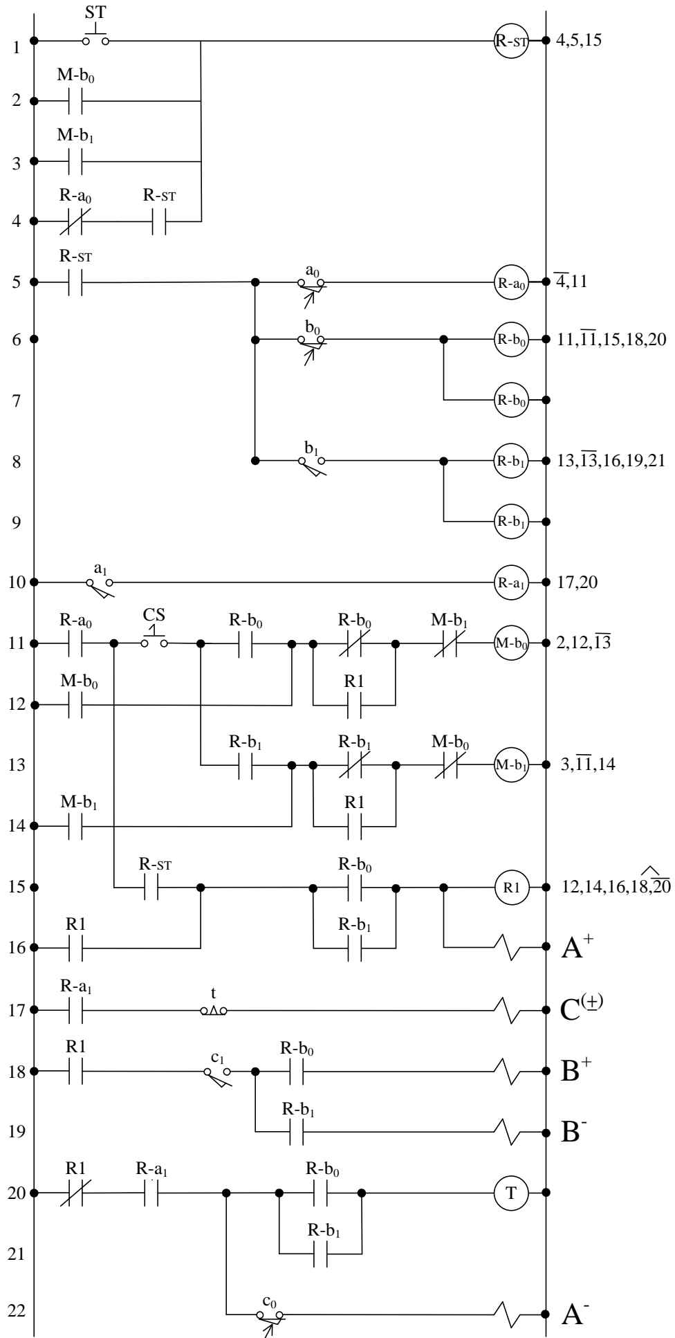
圖8-3 電路圖
