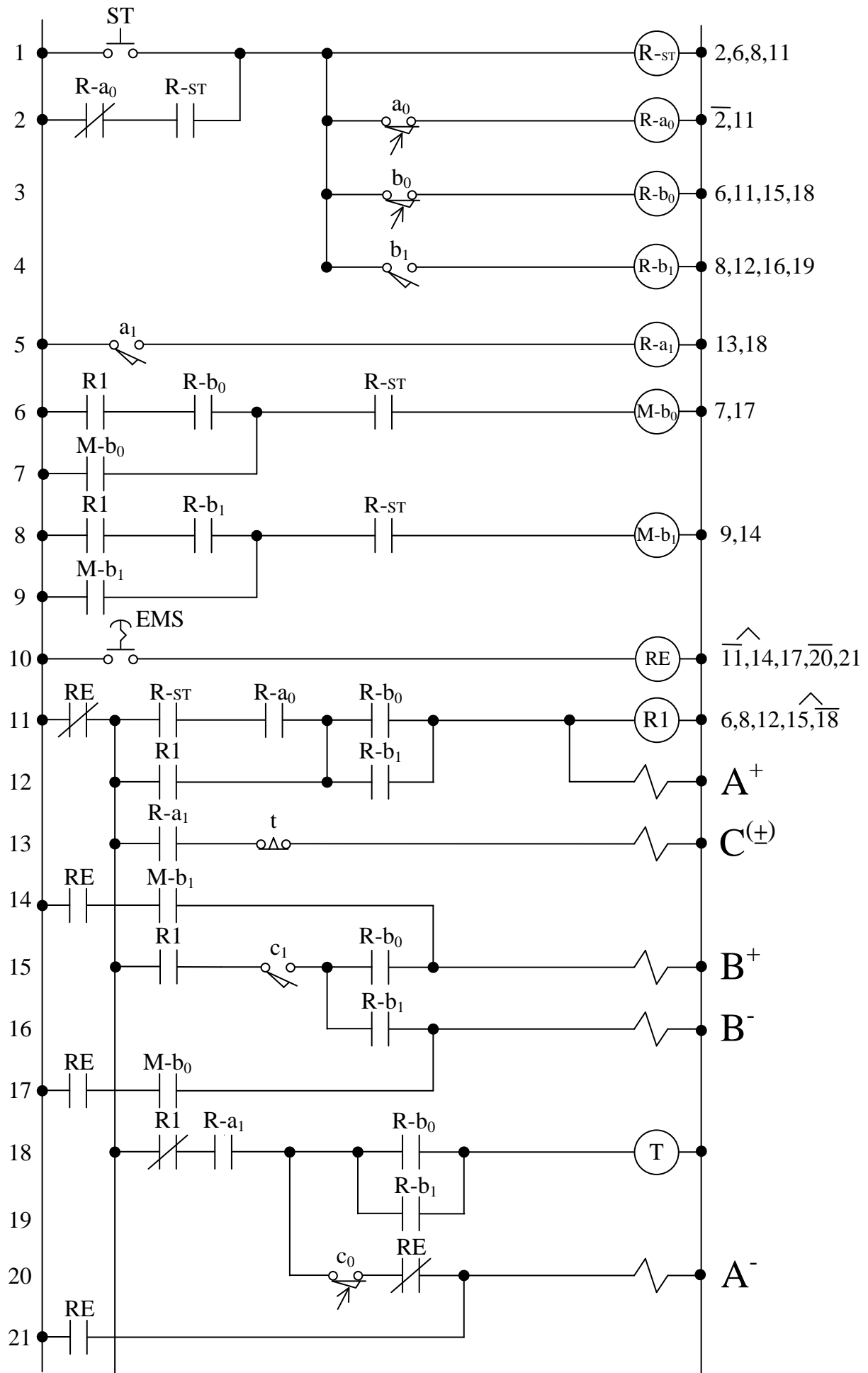
圖7-5a 電路圖
