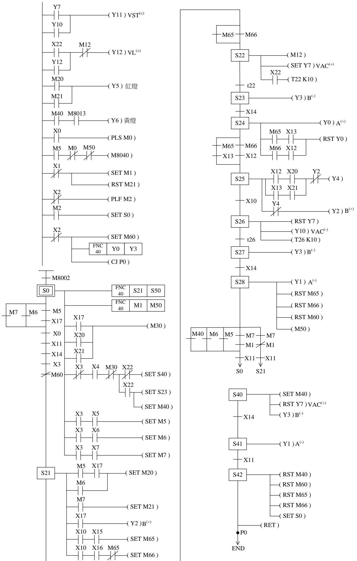
圖4-24 模式a SFC圖
