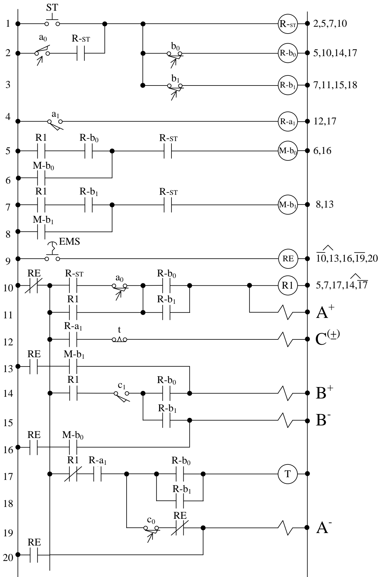
圖7-5b 電路圖(另解)
