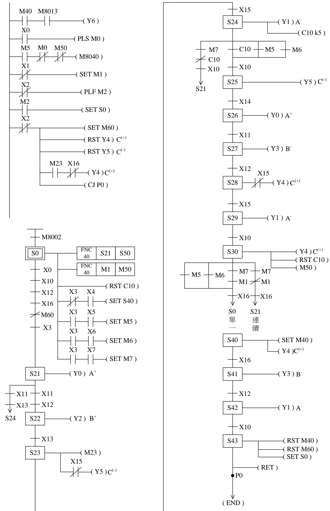
圖 1-22 模式 a SFC 圖
