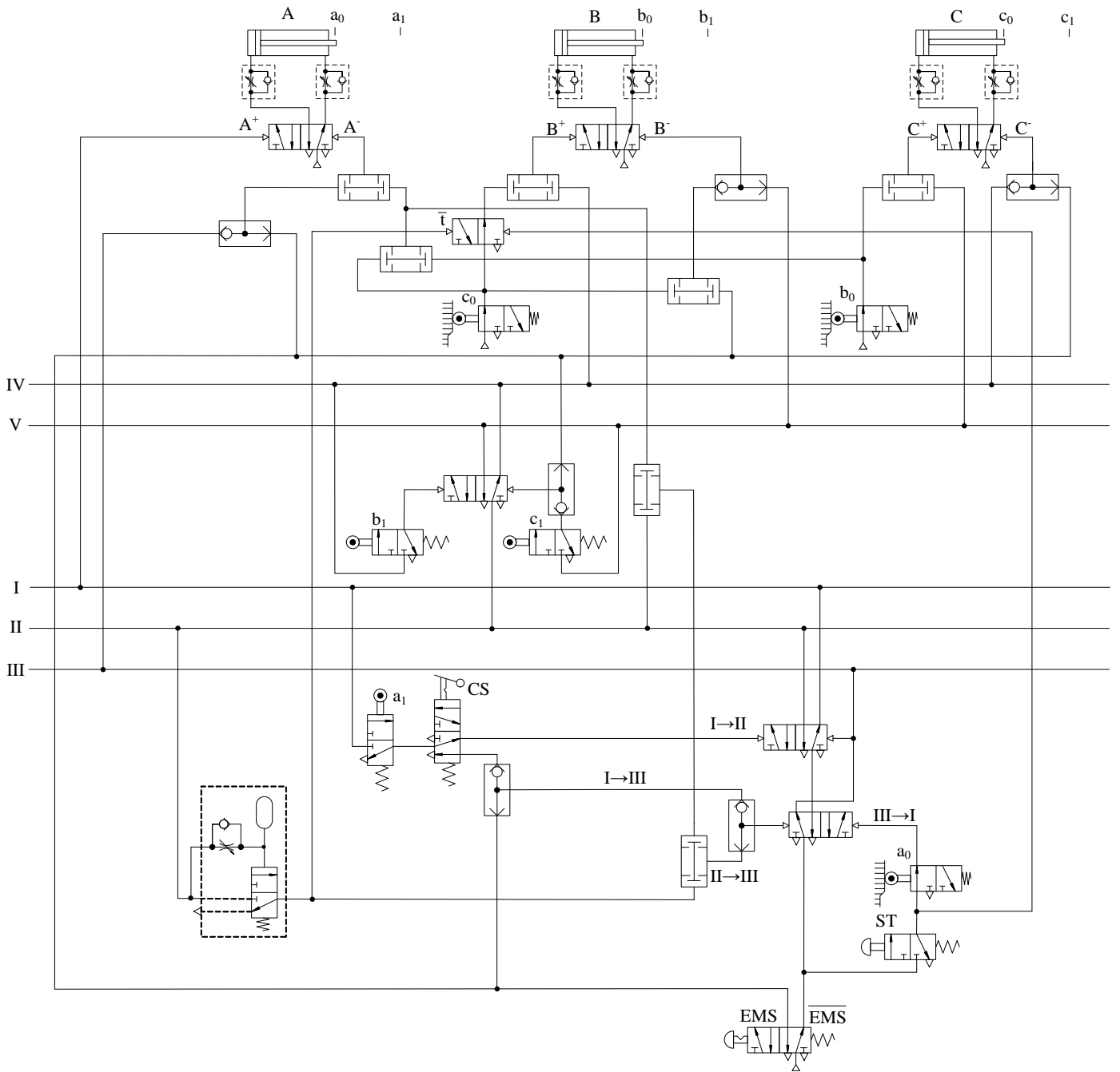
圖10-4 計時反覆動作回路
