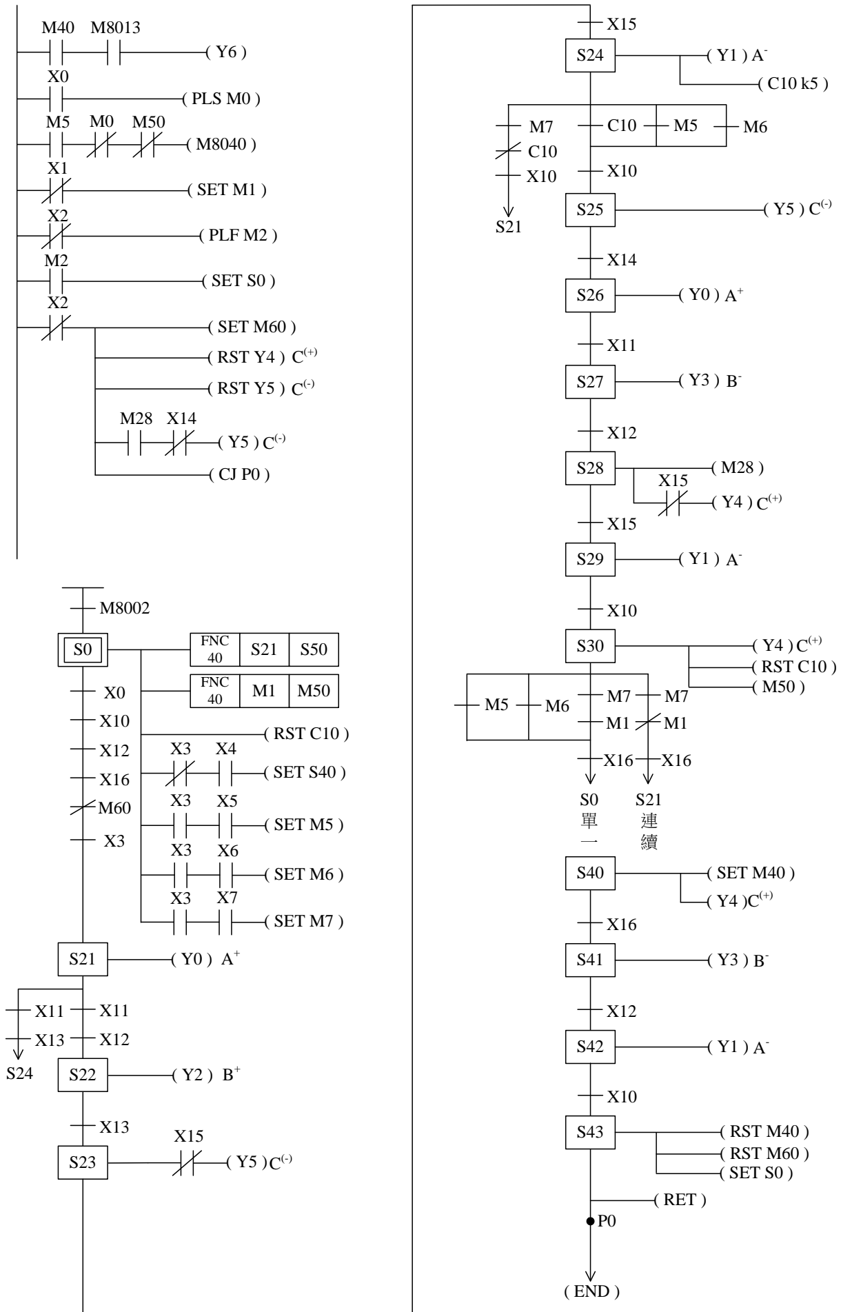
圖 1-44 模式 b SFC 圖
