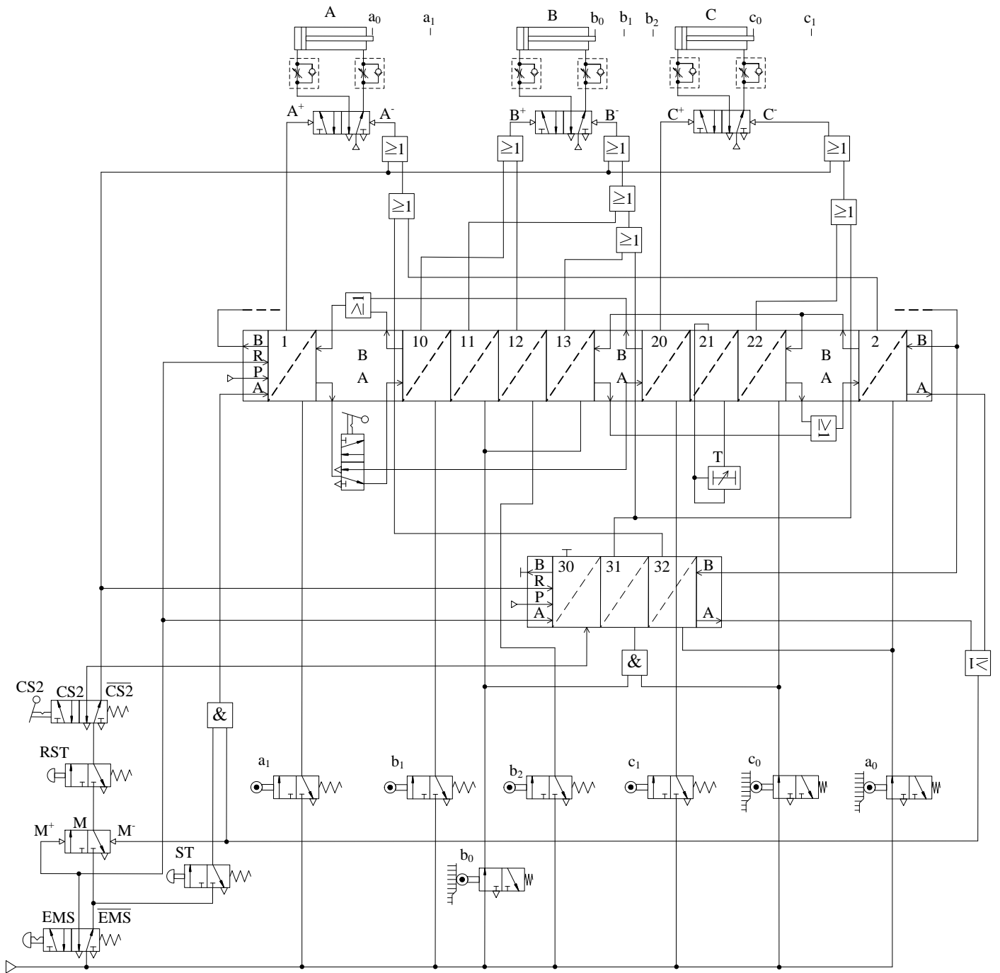
圖 12-8 順序發生器迴路
