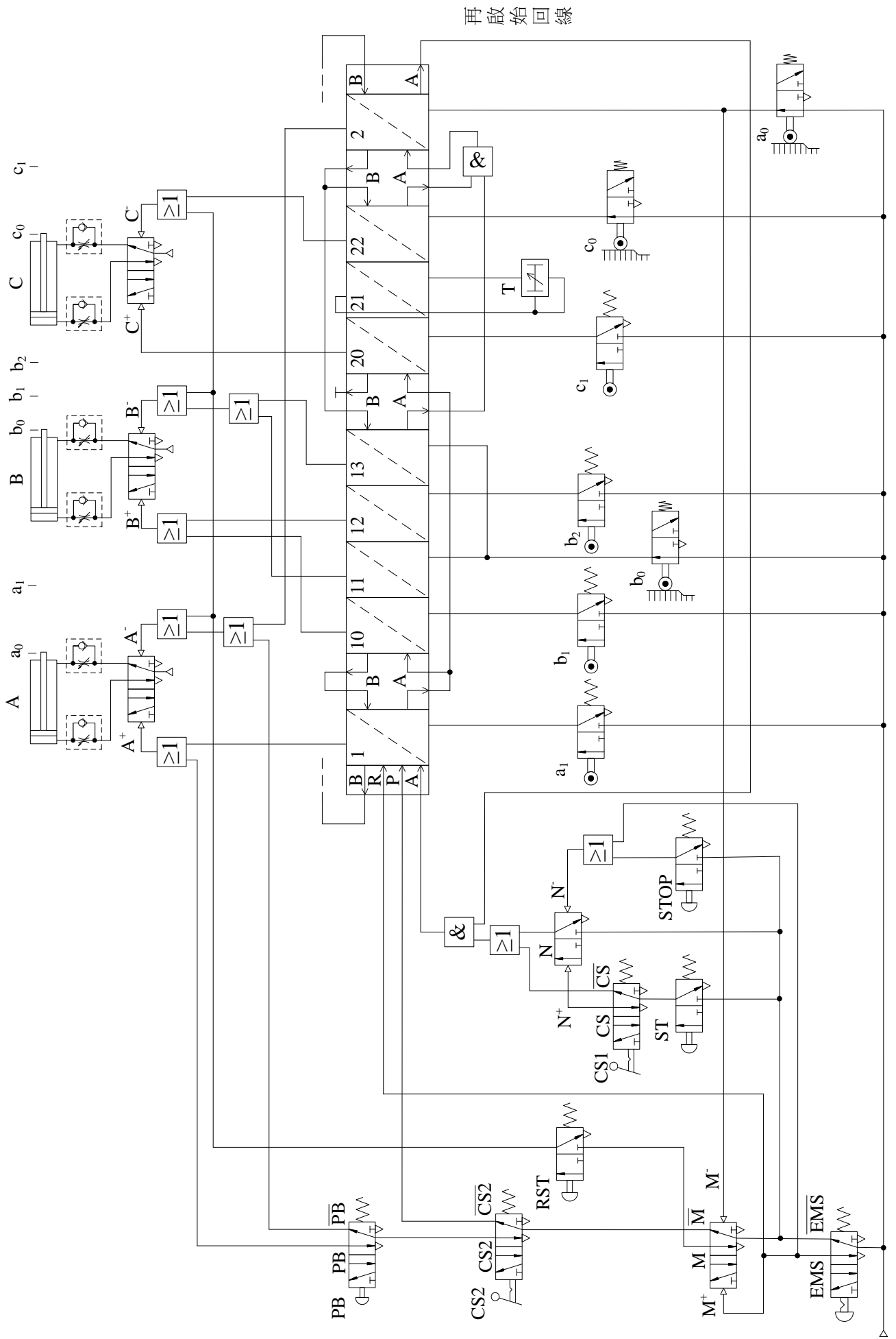
圖11-9 順序發生器迴路
