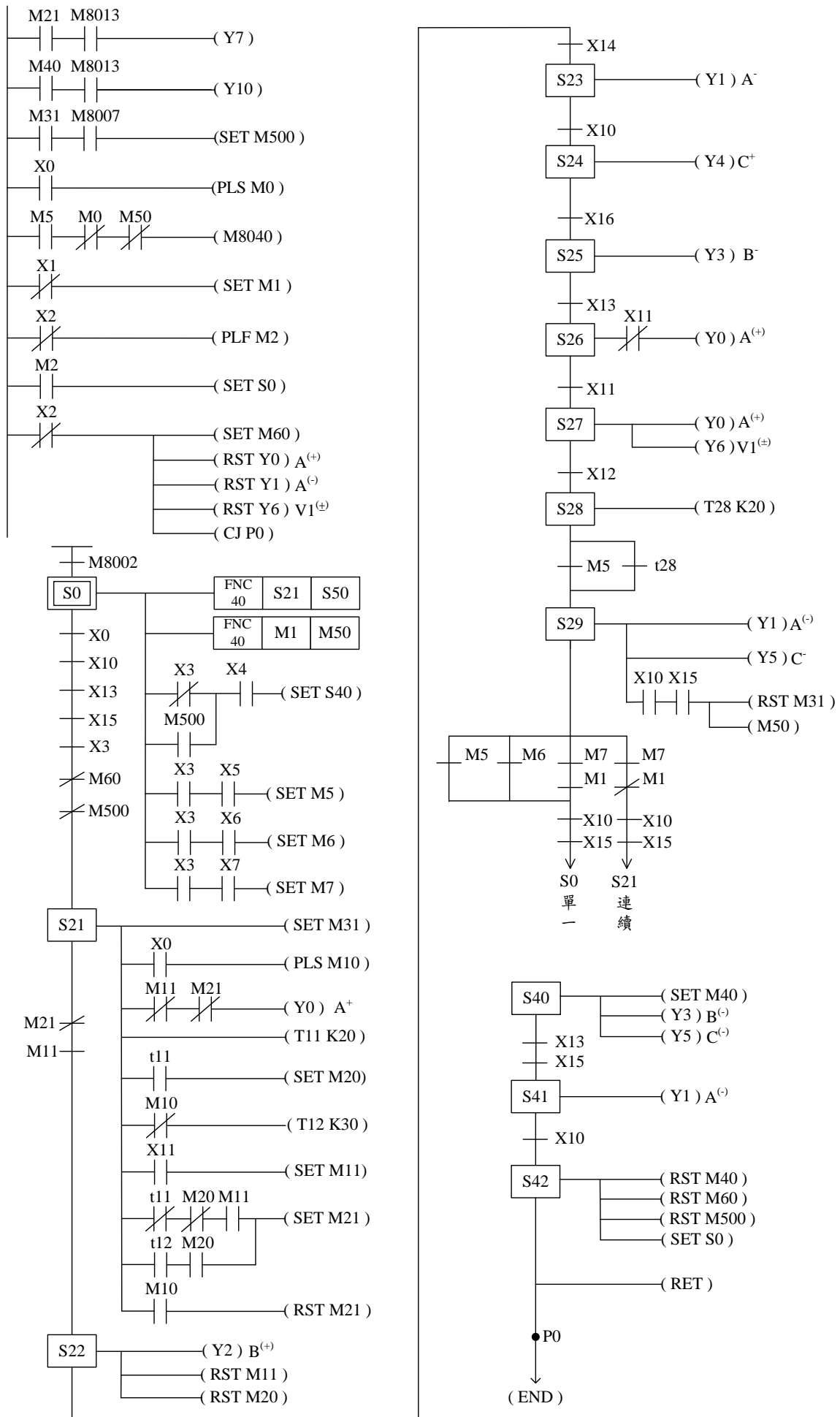
圖5-36 模式b SFC圖
