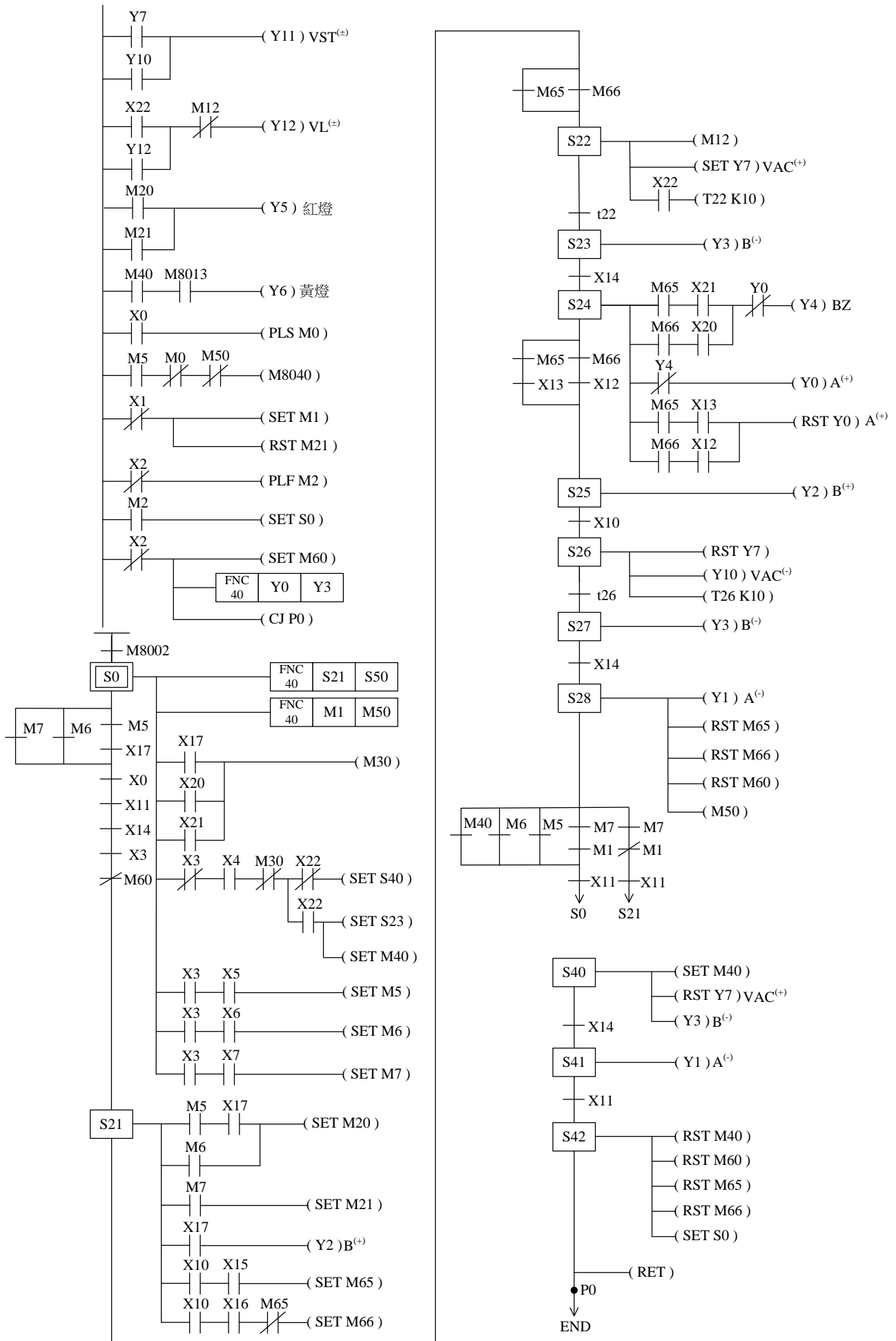
圖3-48 模式b SFC圖
