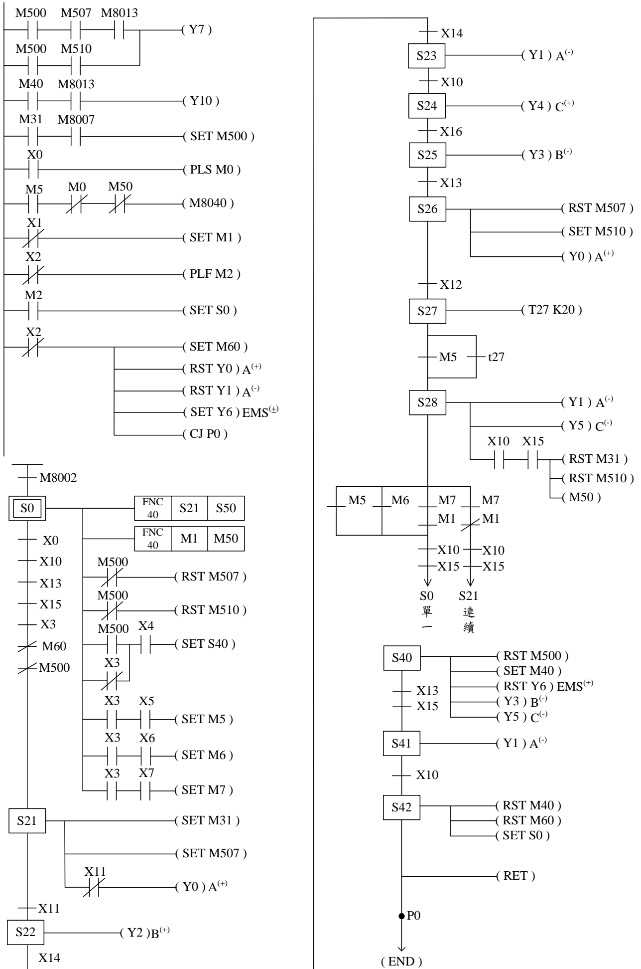
圖6-35 模式b SFC圖
