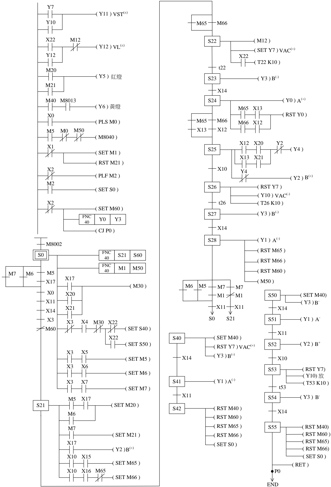
圖4-49 模式b SFC圖
